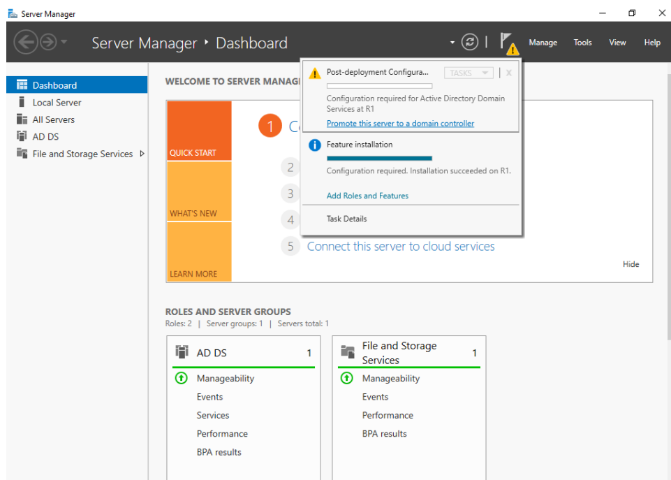
Hình 12-3: Cài Domain
